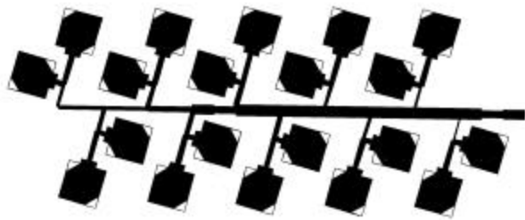
Figure 1 DBS Antenna Subarray
